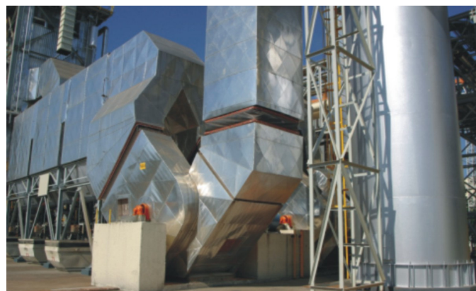
DURATEX – Itapetininga – SP: Exaustores de tiragem induzida da caldeira.
